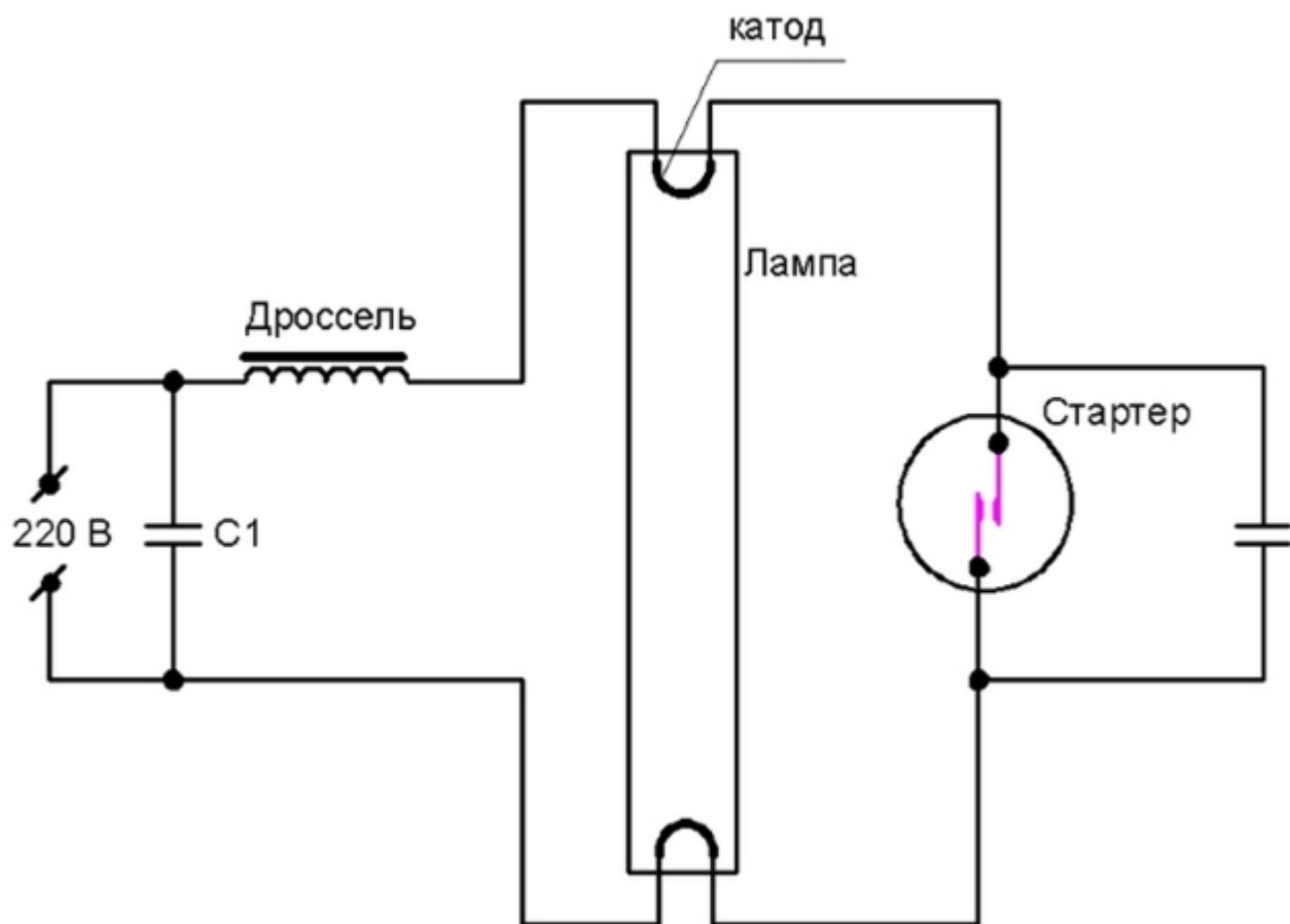
Рис.1. Схема электрическая принципиальная подключения люминесцентной лампы
